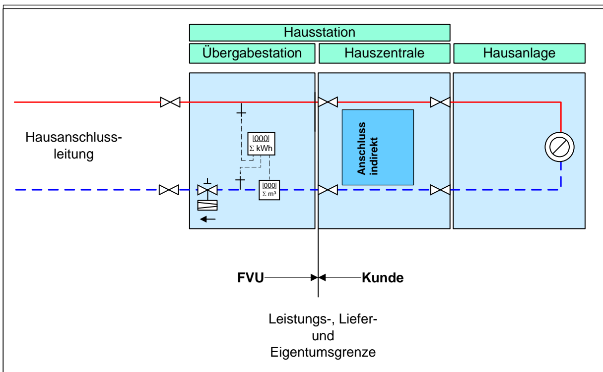
Abbildung 7: Beispiel von Leistungs-, Liefer- und Eigentumsgrenzen
