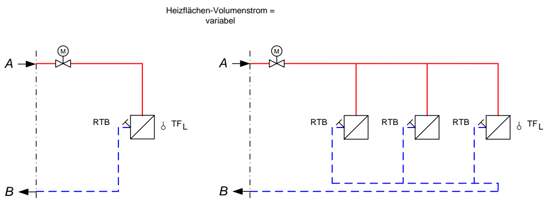
Abbildung 9: Hauszentrale-Raumluftheizung Prinzipschaltbilder für den indirekten Anschluss
