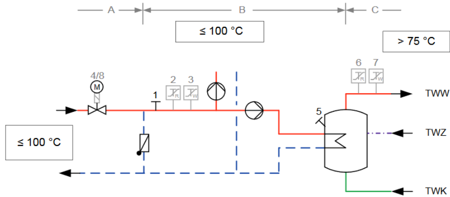
Abbildung zur Tabelle 10: Erforderliche sicherheitstechnische Ausrüstung nach Zeile 3; grau dargestellte Komponenten nicht erforderlich
