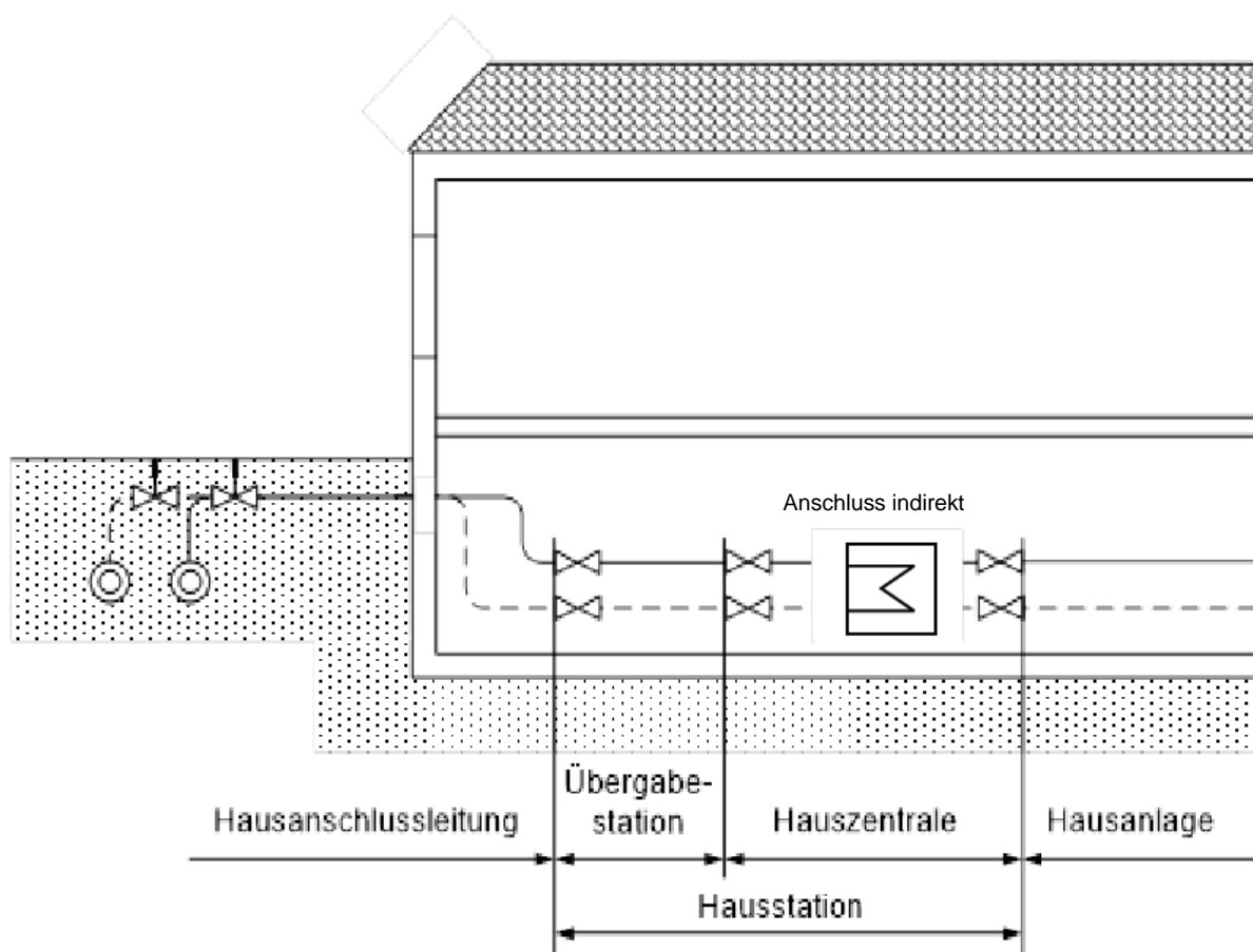
Abbildung 6: Hausanschlussleitung und Hausstation
