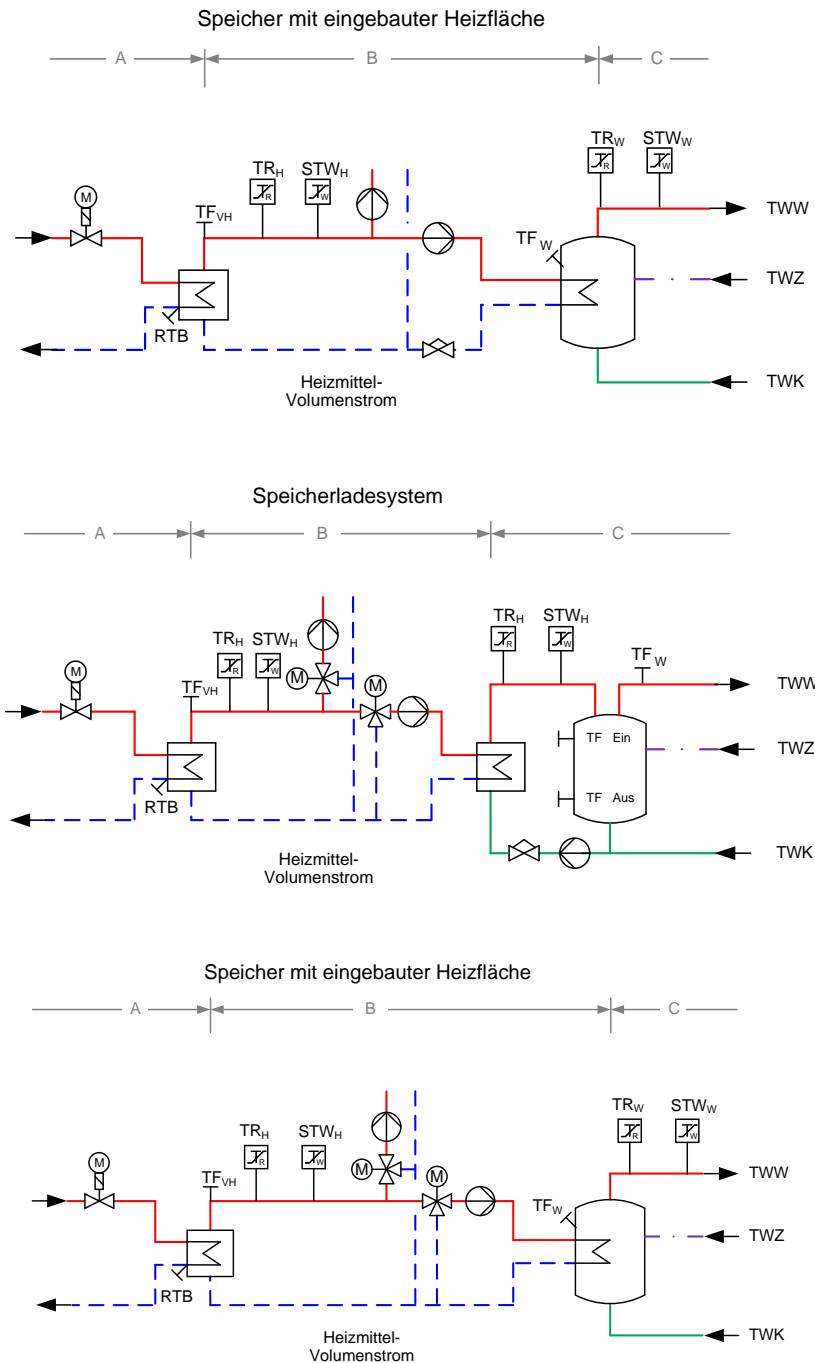
Abbildung 10: Hauszentrale-Trinkwassererwärmung Prinzipschaltbild für den indirekten Anschluss
