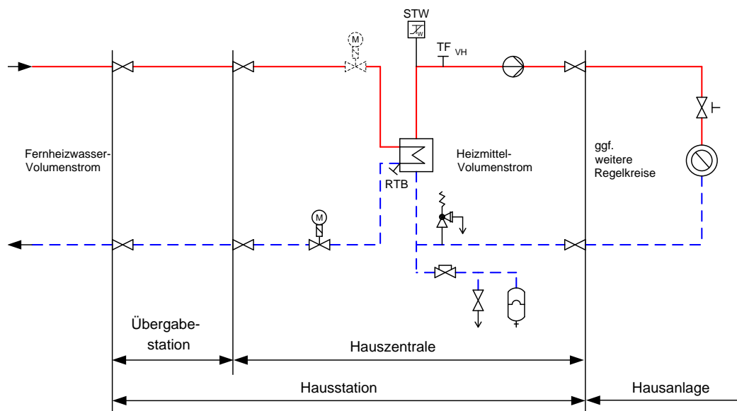
Abbildung 8: Hauszentrale-Raumheizung-Prinzipschaltbild für den indirekten Anschluss
