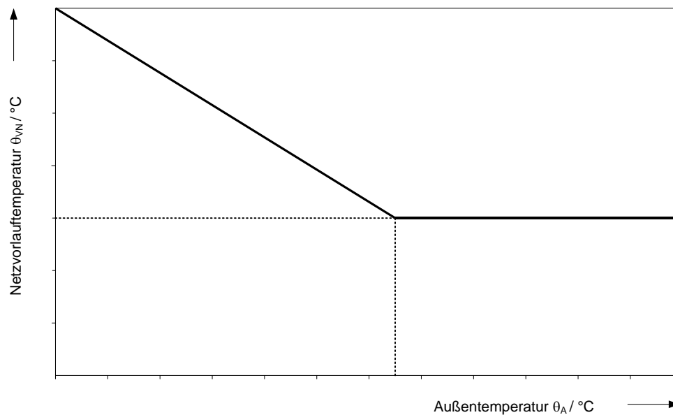
Abbildung 1: Netzvorlauftemperatur \theta_{VN} in Abhängigkeit von der Außentemperatur \theta_A ; prinzipieller Verlauf einer gleitend-konstanten Fahrweise (evb)
